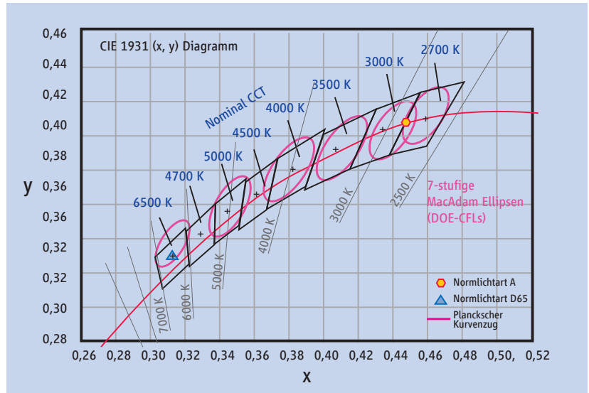
Abb. 8: Standard-Binningstruktur gemäß ANSI C78.377A als Ausschnitt aus dem CIE-Farbdreieck
