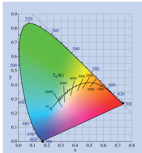
Abb. 5: CIE Normvalenzsystem-Koordinatensystem zur Definition aller durch den Menschen wahrnehmbaren Farben
