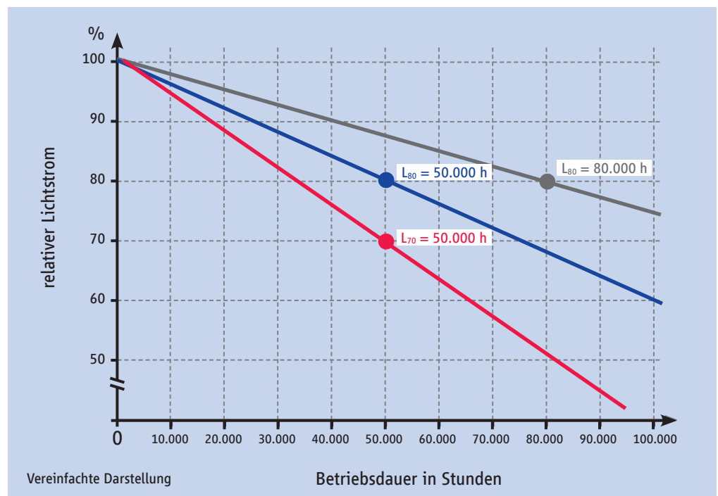
Abb. 13: Schematische Darstellung des Lichtstromverlaufs über der Betriebszeit
