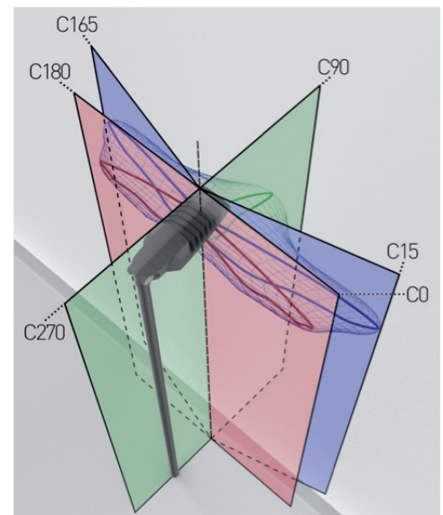
Abb. 4: Beispiel der Lichtstärkeverteilung einer Straßenleuchte
