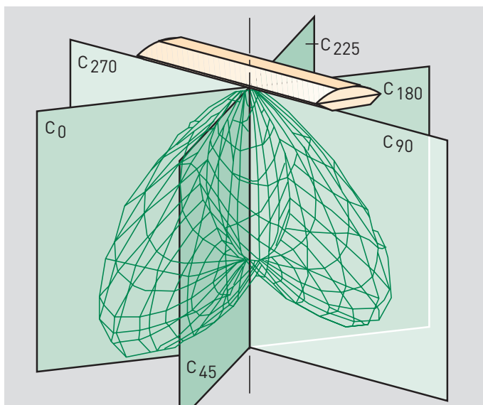
Abb. 3: Beispiel der Lichtstärkeverteilung einer Innenraumleuchte
