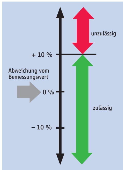
Abb. 1: Darstellung der Toleranzfelder der Bemessungseingangsleistung
