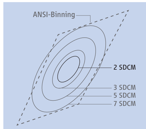
Abb. 10: MacAdam-Ellipsen innerhalb eines ANSI-Binnings
