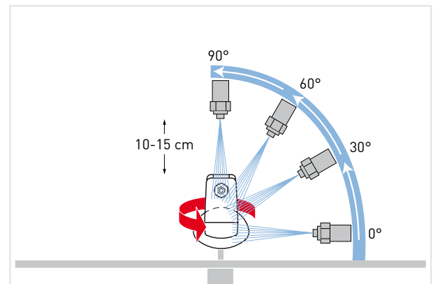
> Schematische Darstellung der Schutzartprüfung IP 69K
