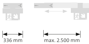
Modul mit Rettungswegkennzeichnung verschiebbar
