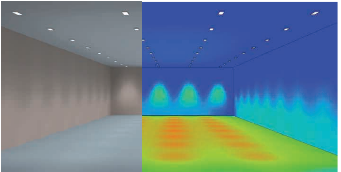
Beleuchtungsstärke (lx)
